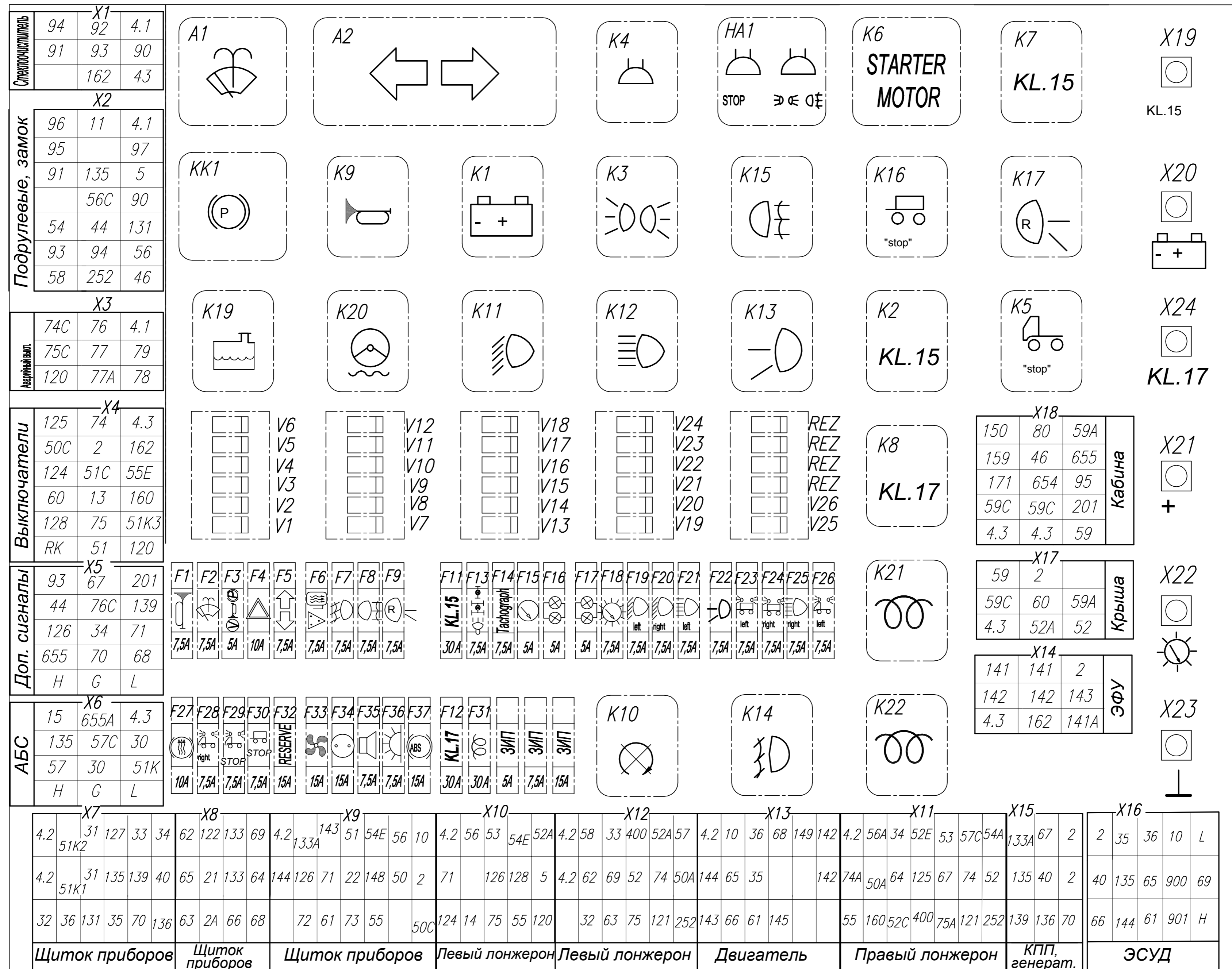
Табличка расположения элементов БКА-4М ОДО "Павезж" (Приложение 2.3)
